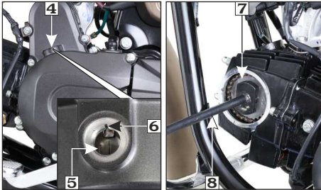
(4) टाइमिंग होल कैप (5) 'T' मार्क (6) इंडेक्स मार्क (7) कैम स्प्रॉकेट (8) स्पेशल टूल
