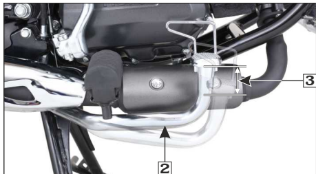
(2) इंटीग्रेटेड/रियर ब्रेक पेडल (3) फ्री प्ले 20-30 mm
