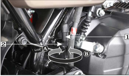
(1) स्टॉप लैंप स्विच (A) एडवांस
