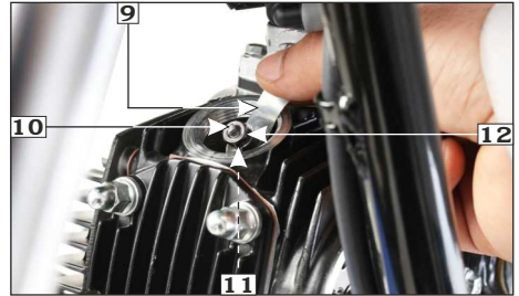
(9) फीलर गेज (11) वाल्व स्टेम
