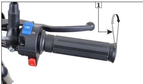
(1) फ्री प्ले : 2-6 mm
