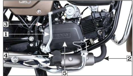
(1) किक स्टार्टर पेडल
