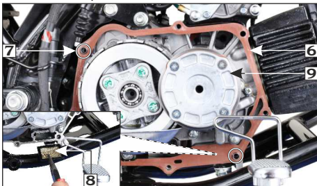
(6) गैस्केट (7) डॉवेल पिन्स (8) ऑयल फिल्टर स्क्रीन (9) सेन्ट्रीफ्यूगल फिल्टर कवर
