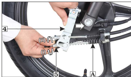
(4) इंटीग्रेटेड ब्रेक आर्म (5) पहला एडजस्टर नट (i) फ्री प्ले कम करना (ii) फ्री प्ले बढ़ाना
