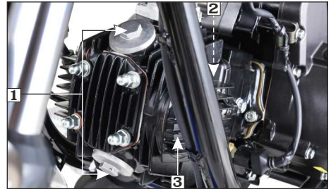
(1) टैपेट कवर्स
